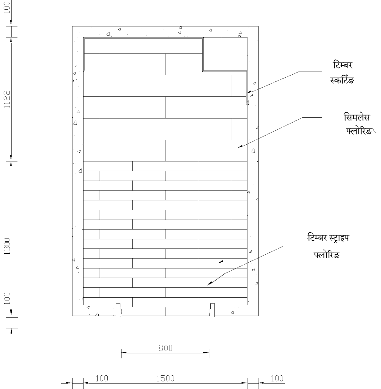
लेआउट प्लान
