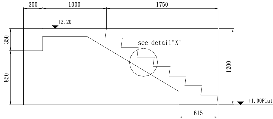
सेक्शनल भ्यू A-A SECTIONAL VIEW A-A
