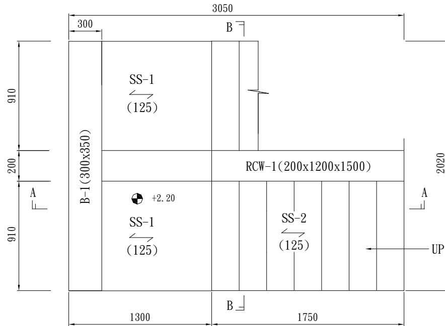
खण्ड B-B (1:30) PLAN VIEW प्लान भ्यू
