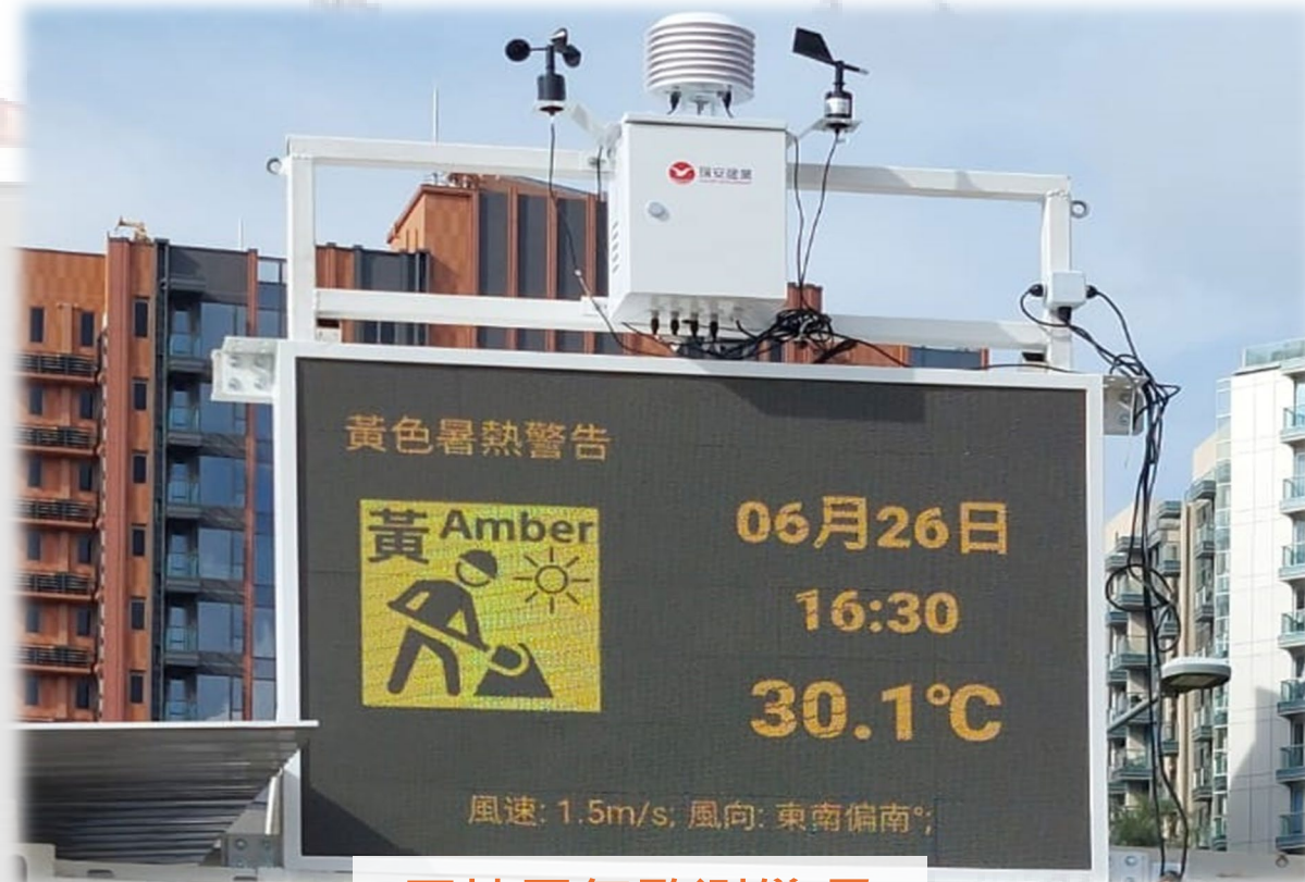
工地天氣監測儀 及 天氣資訊顯示屏
