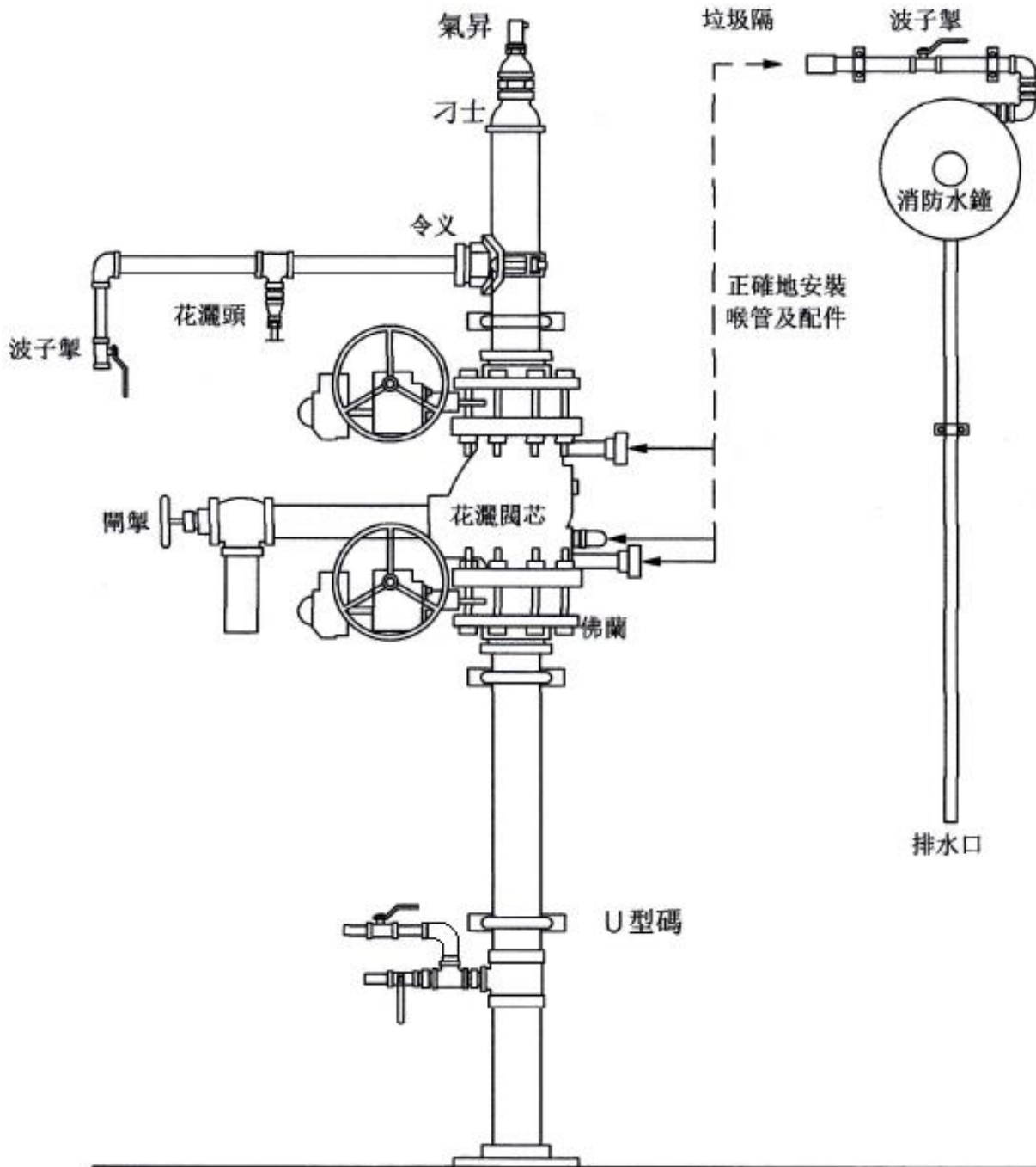
安裝花灑閥芯喉管
