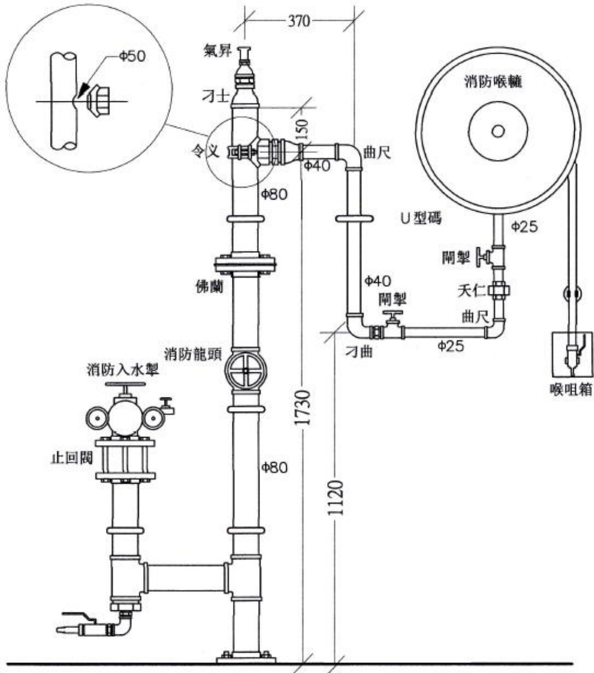
安裝消防龍頭及接駁消防喉轆
