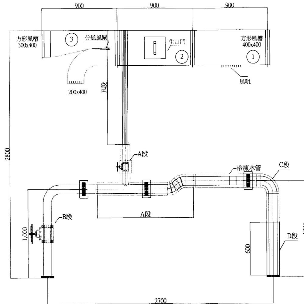
風槽及保溫施工立面圖
