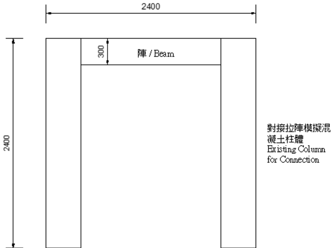
立面圖 Front Elevation
