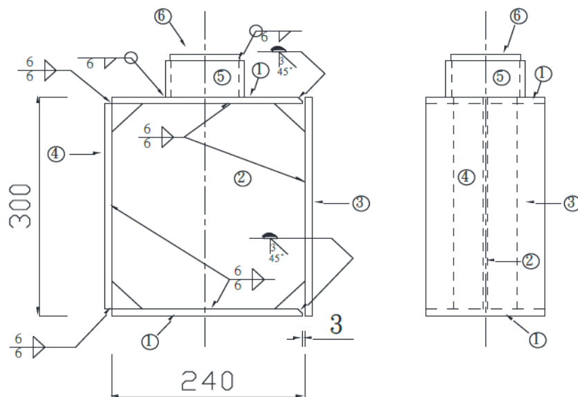
視圖 A-A
