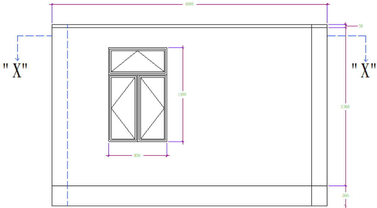
立面圖
