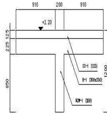
سیکشنل ویو B-B SECTIONAL VIEW B-B
