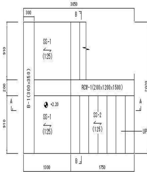
پلان ویو PLAN VIEW
