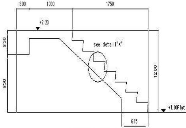
سیکشنل ویو A-A SECTIONAL VIEW A-A
