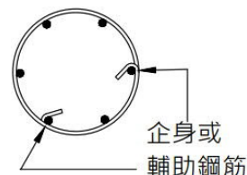
圓洛細節圖
