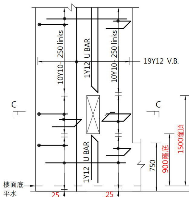
W1 間牆鋼筋結構正視圖
