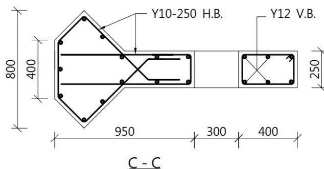
W2 間牆鋼筋結構平面圖
