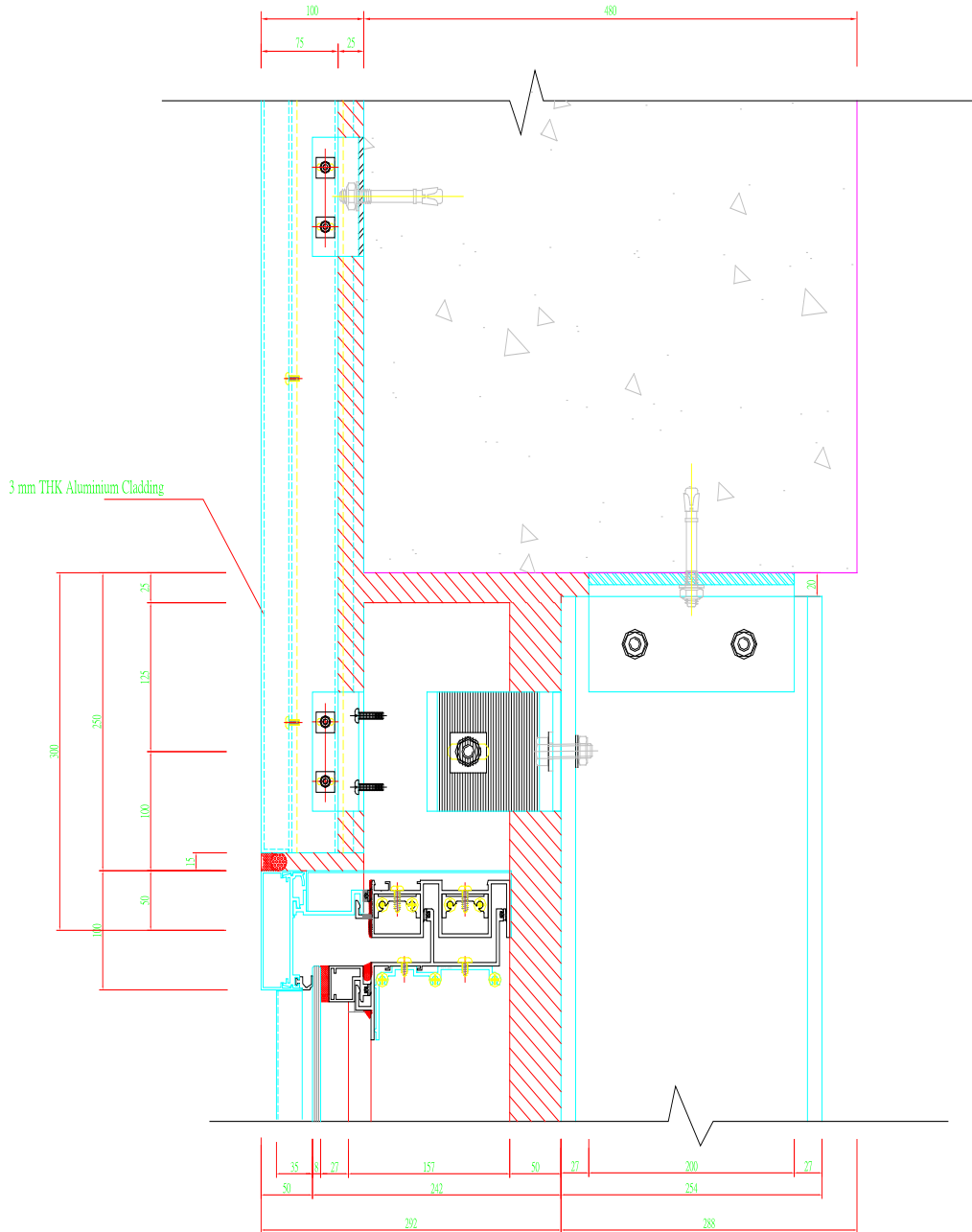
क्रस सेक्शन A
