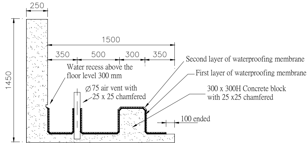
Sec A-A
