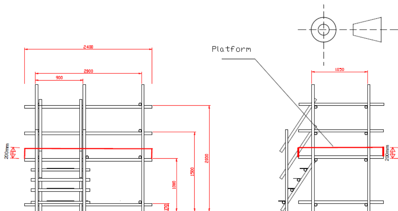
金屬棚架圖片 (只供參考)
