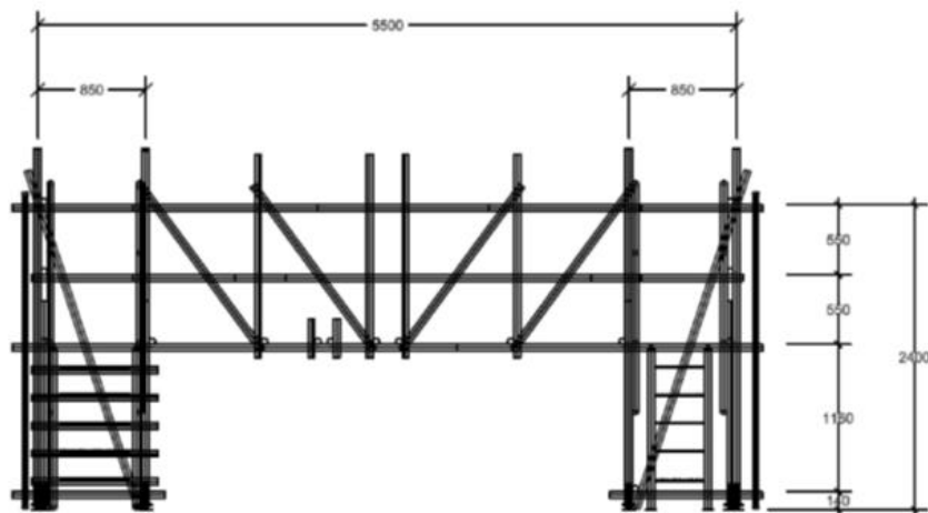
側視圖 — 正面
