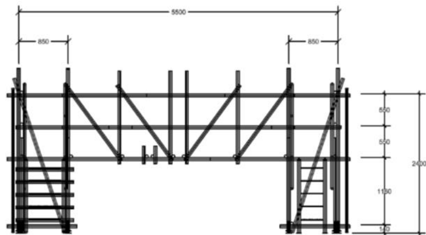
側視圖 - 正面
