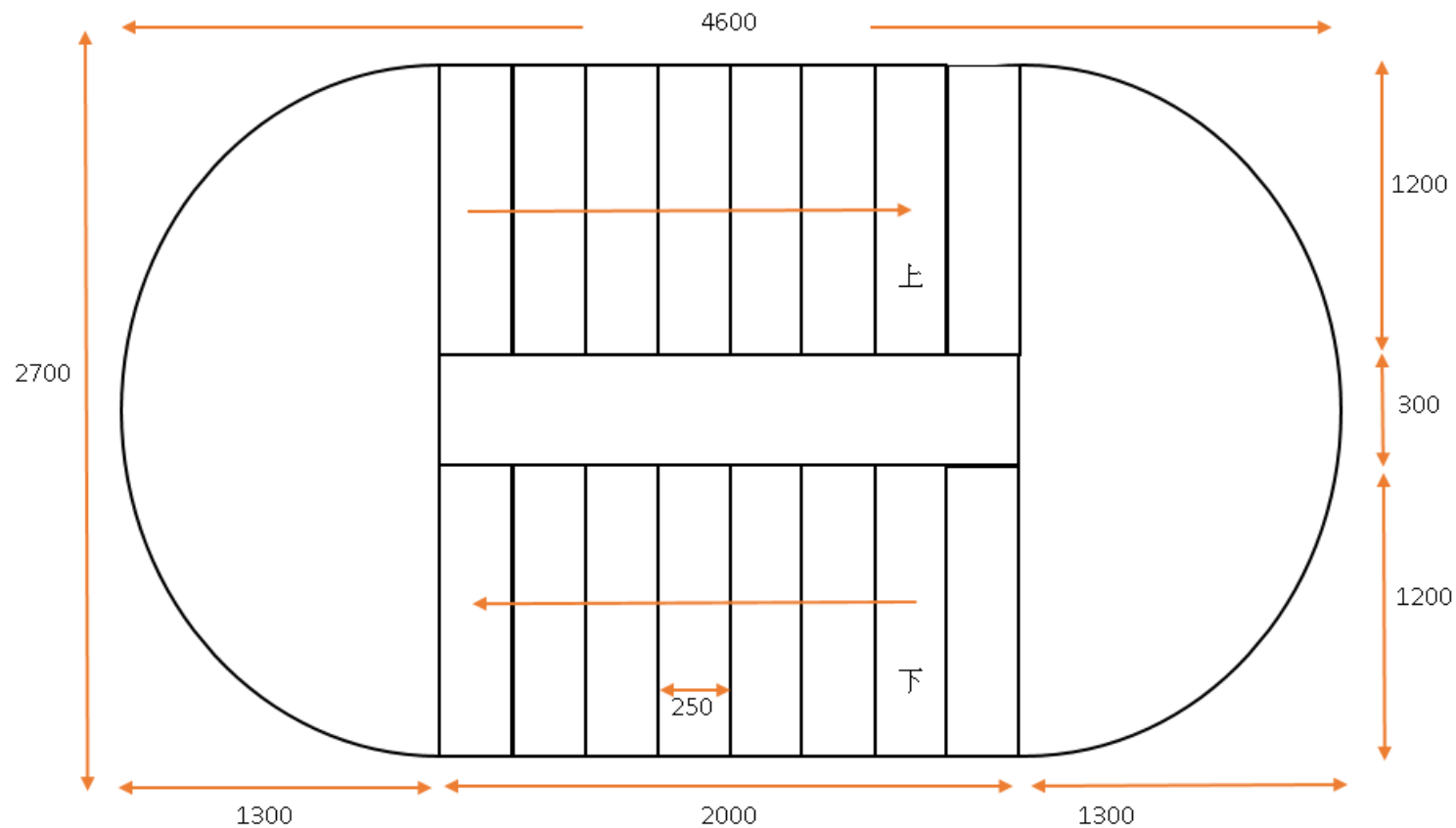
平面圖
