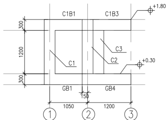
立面圖
