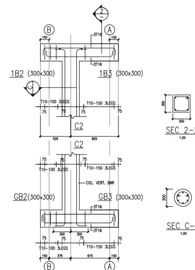
樑柱鋼筋大樣圖
