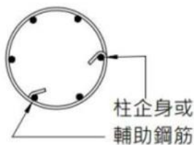
圓柱洛細節圖
