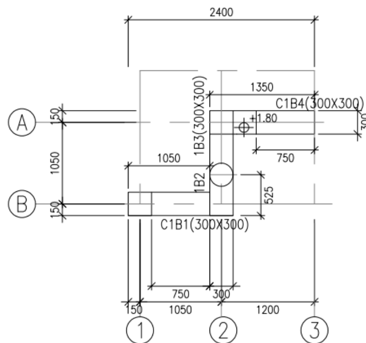
1/F 平面佈置圖
