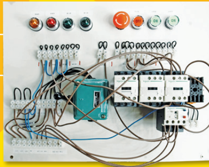
【中】星角起動器 【英】Star-delta Starter
