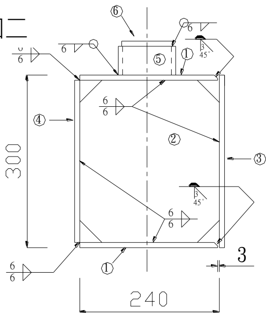
視圖 A-A
