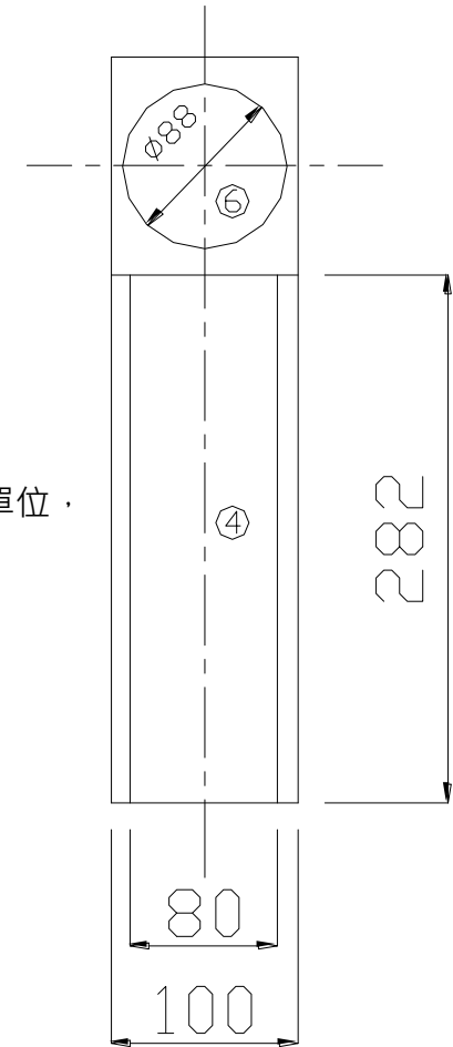
平面圖
