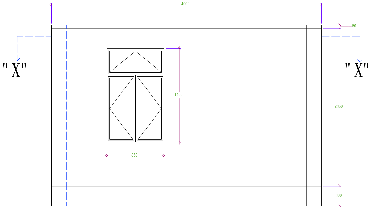
立面圖
