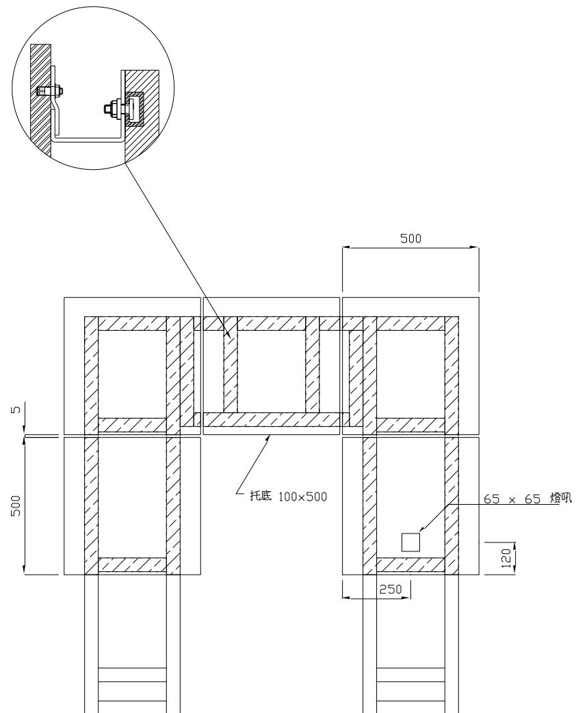
正面圖
