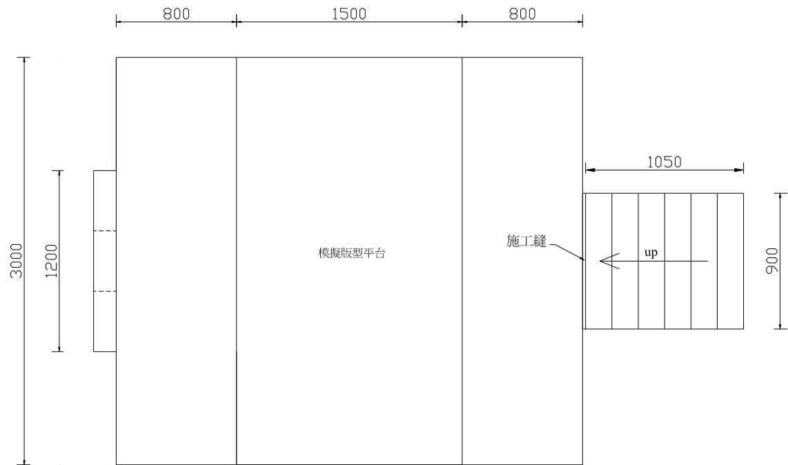
平面圖
