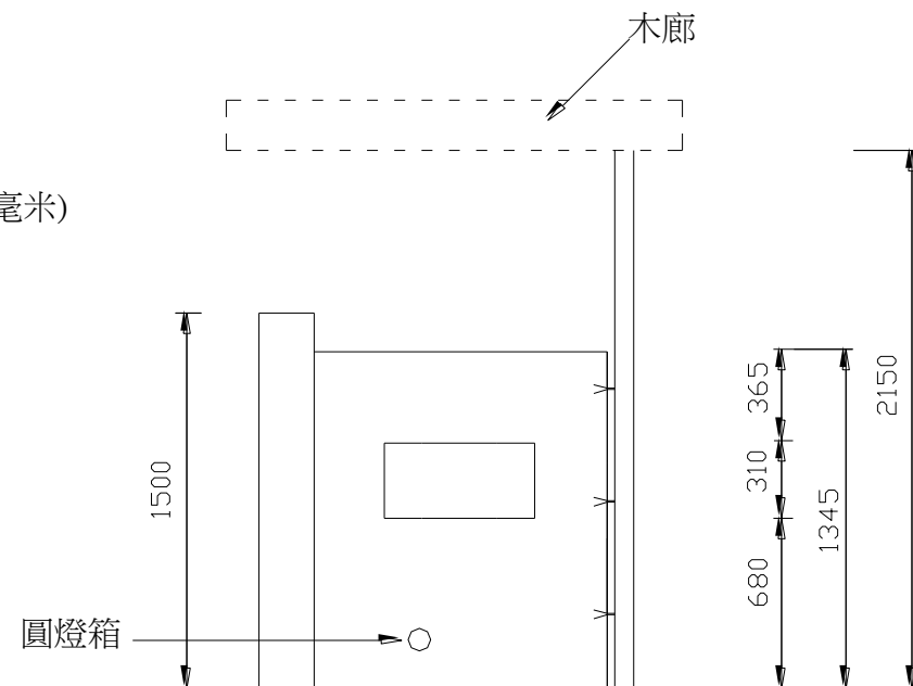
正面圖
