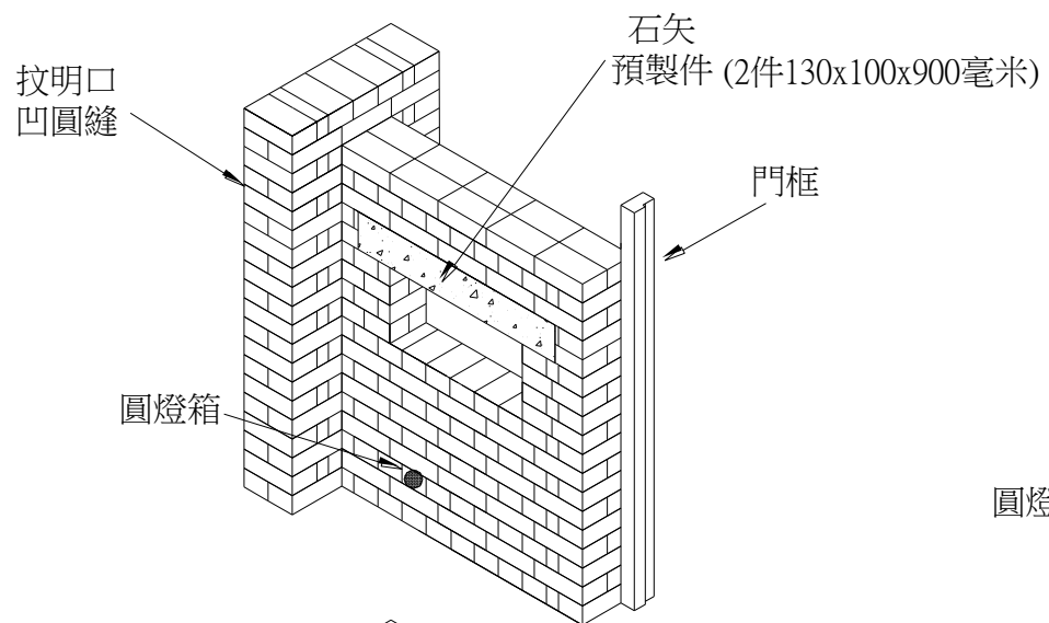
立體圖
