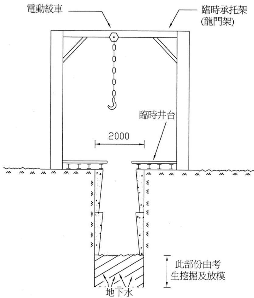
正剖面圖
