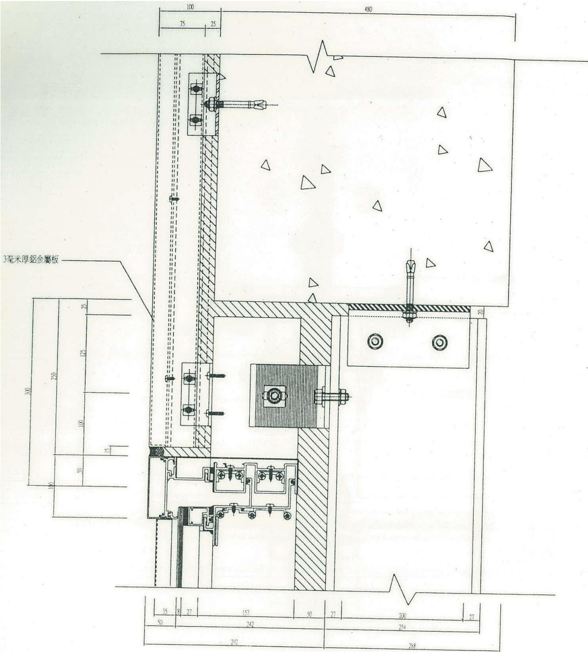
剖面圖 A
