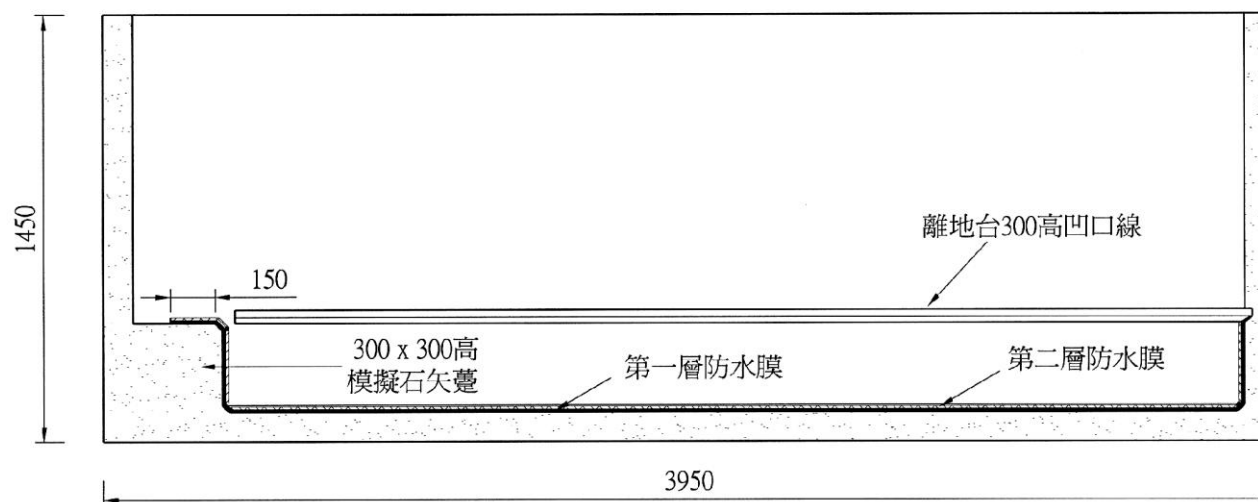
剖面圖 C
