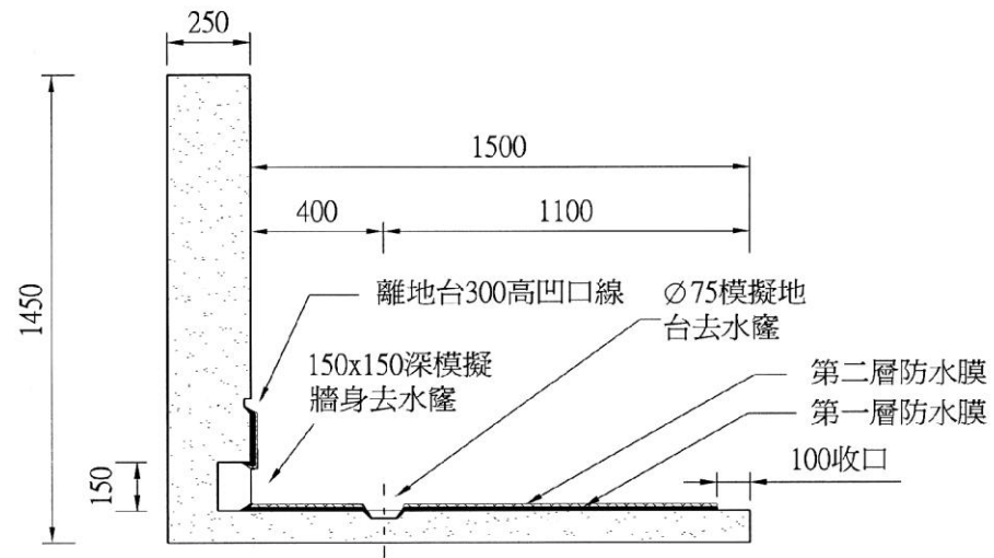
剖面圖 B
