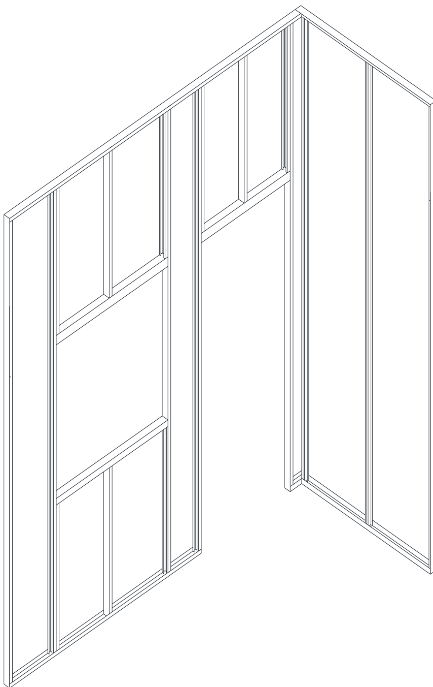
間隔(金屬骨架)工施工圖一 (金屬鐵框架組裝圖)
