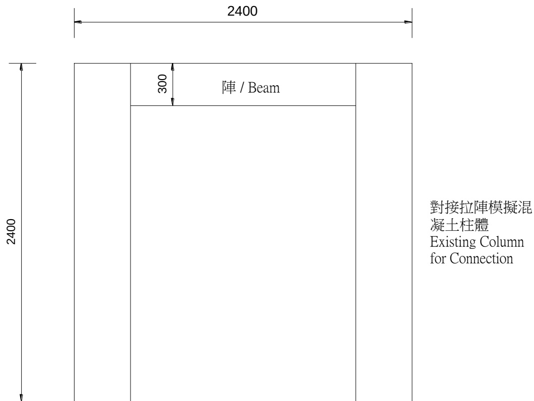
立面圖 Front Elevation
