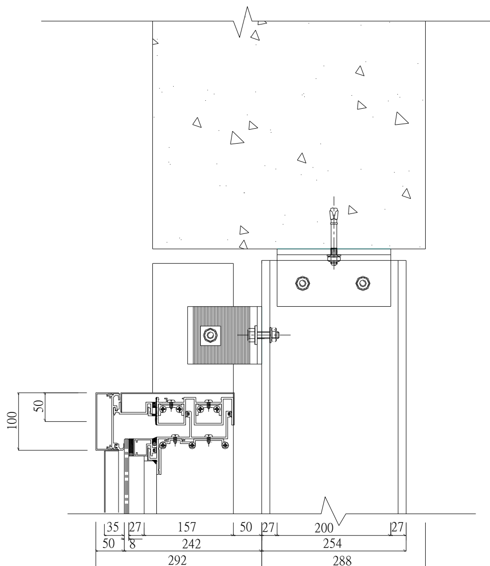
剖面圖 A
