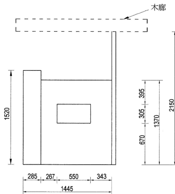
平面圖
